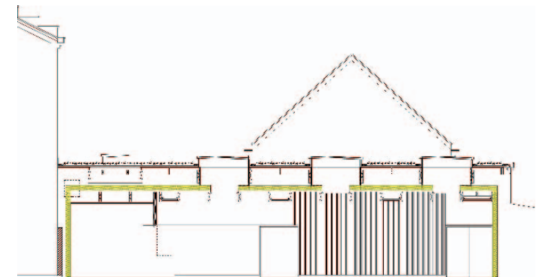
Coupe longitudinale révélant le système de la « boîte dans la boîte ».
